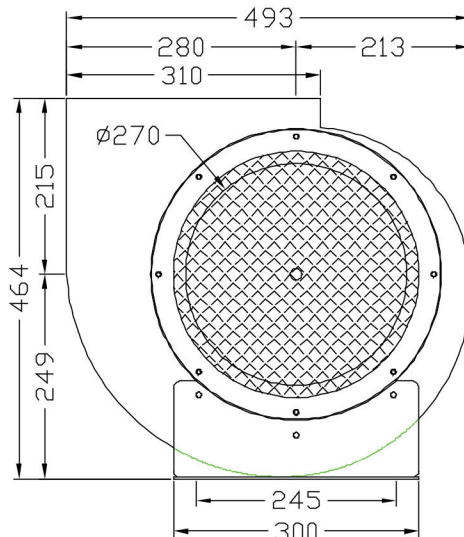
上視圖 (Top View)
