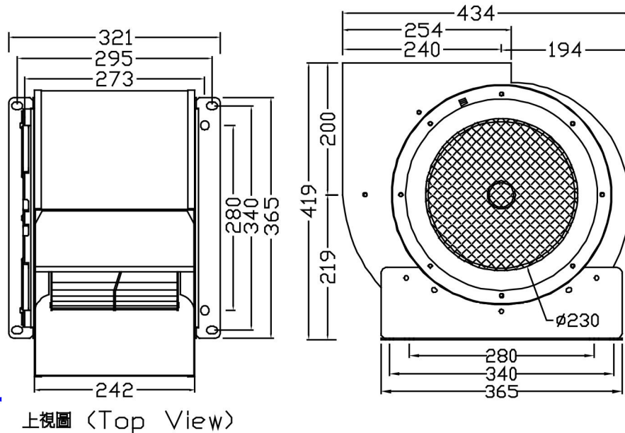
可變換3速/3 Speed motor
