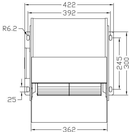
上視圖 (Top View)
